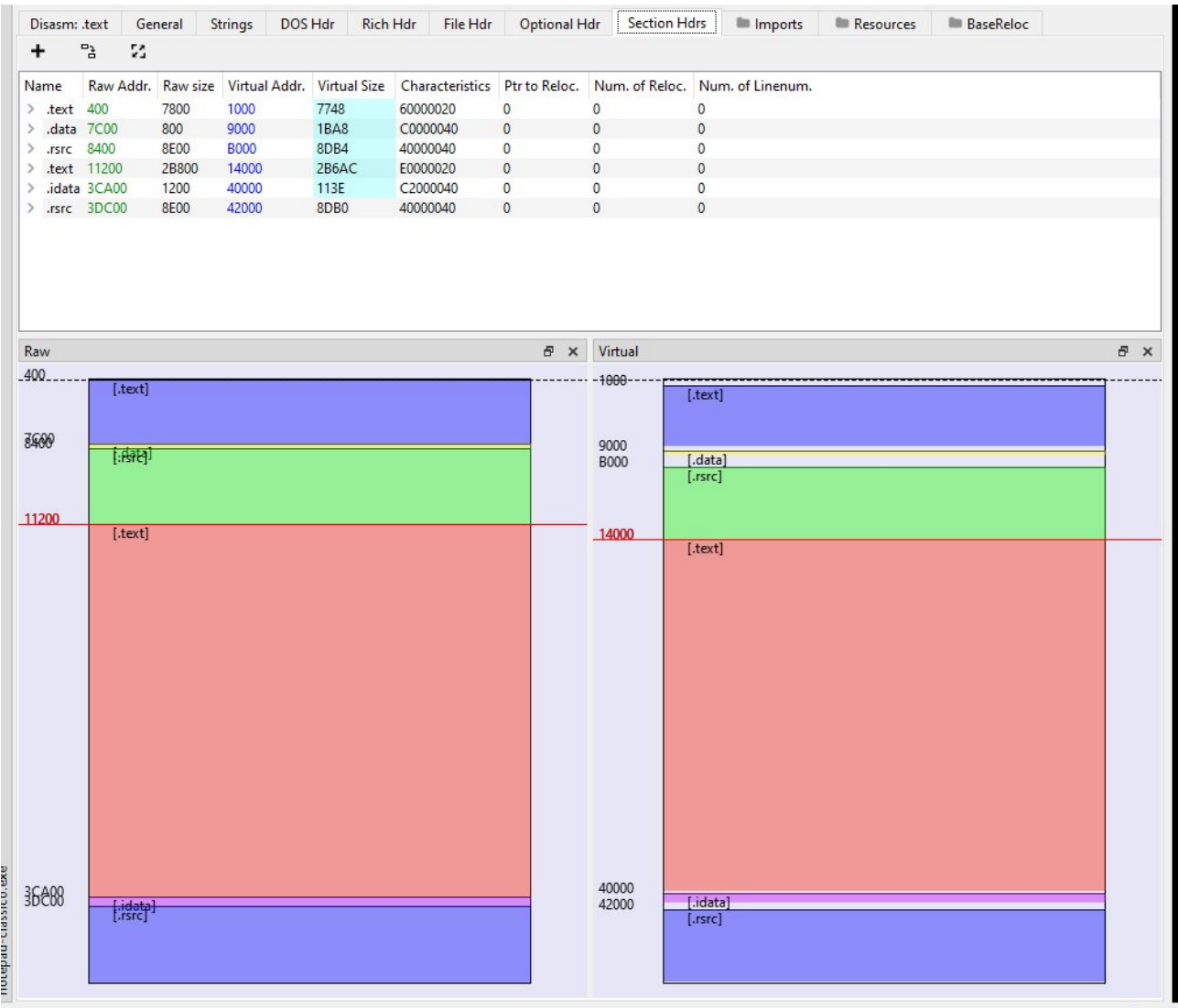
Fig. 2 — Tab Section Hdrs PE-bear: 6 sezioni con layout Raw e Virtual. La seconda .text (rosa) domina lo spazio.
