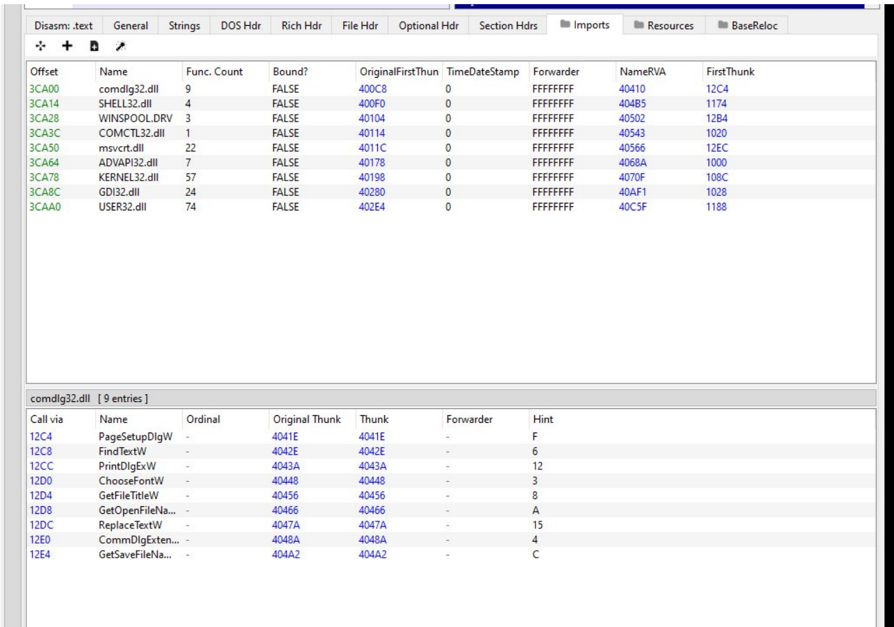
Fig. 1 — Tab Imports PE-bear: 9 DLL con conteggio funzioni e dettaglio comdlg32.dll.
